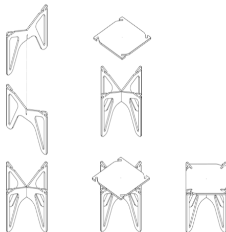
Figura 5 – Modo de montagem do banco em três passos
