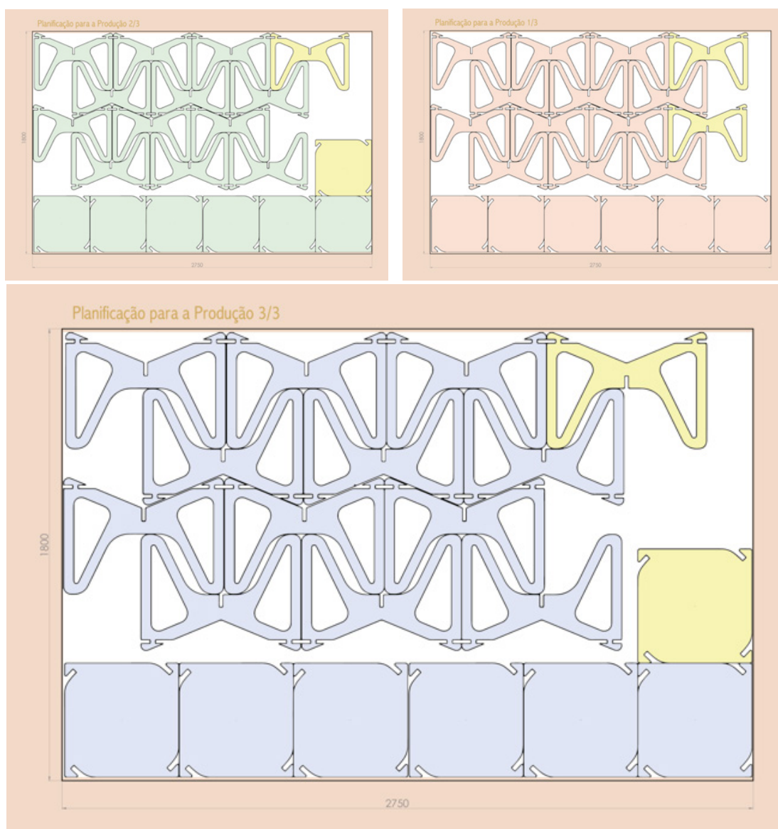
Figura 6 – Planejamento da produção do desenho técnico para o melhor aproveitamento das placas de MDF. A cada três placas, podem ser produzidos 20 bancos
