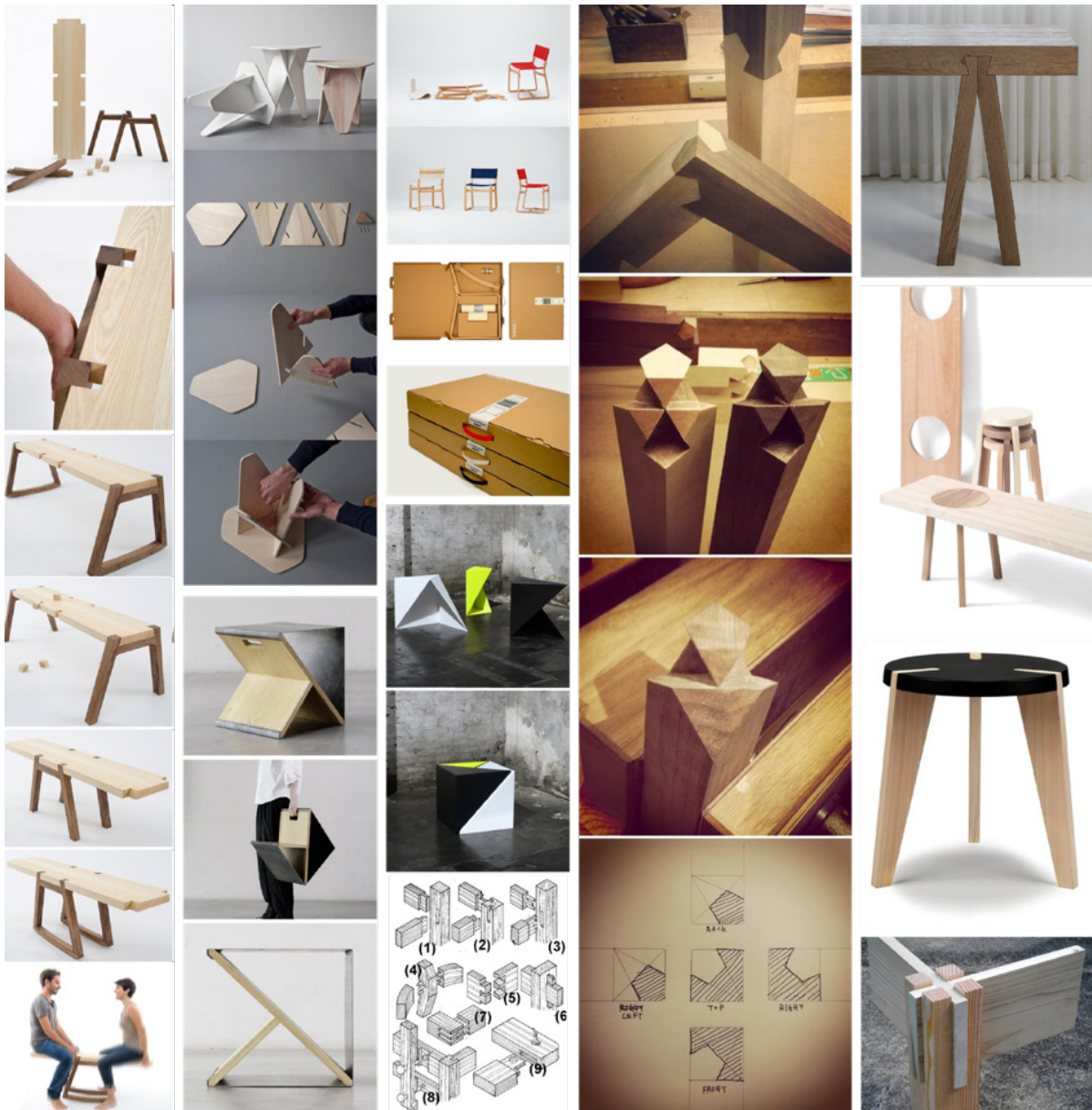
Figura 2 – Moodboard com produtos similares e componentes de mobiliário para o projeto
