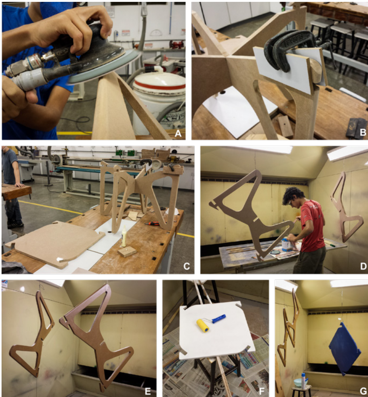
Figura 8 – Processo de acabamento do protótipo do banco Catraca. Lixamento das pernas (A); reparos e montagem (B e C); acabamento com verniz nas pernas do banco (D e E); pintura do assento com primer e tinta azul (F e G)
